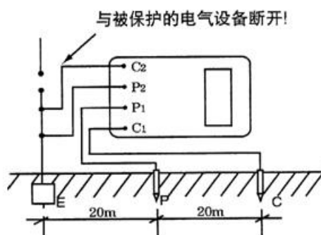
图 6 地桩法测量
