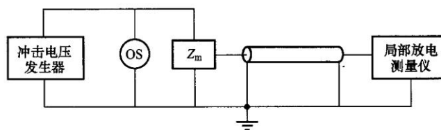
图4 测量阻抗过电压保护性能测试接线图
